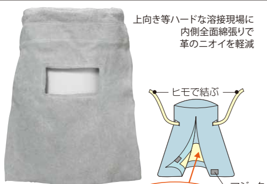
MET-1 床革頭巾 ■サイズ：頭周 66cm・長さ 38cm
