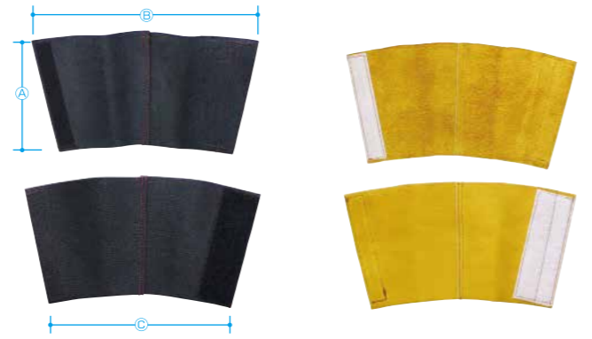
SL-20 床革腕カバー ■サイズ：長さ 50cm・上部腕周 47cm 袖口周 32cm 【1双組】 BR-SL2507 茶床革腕カバー
